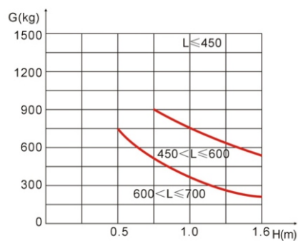
负载曲线图
